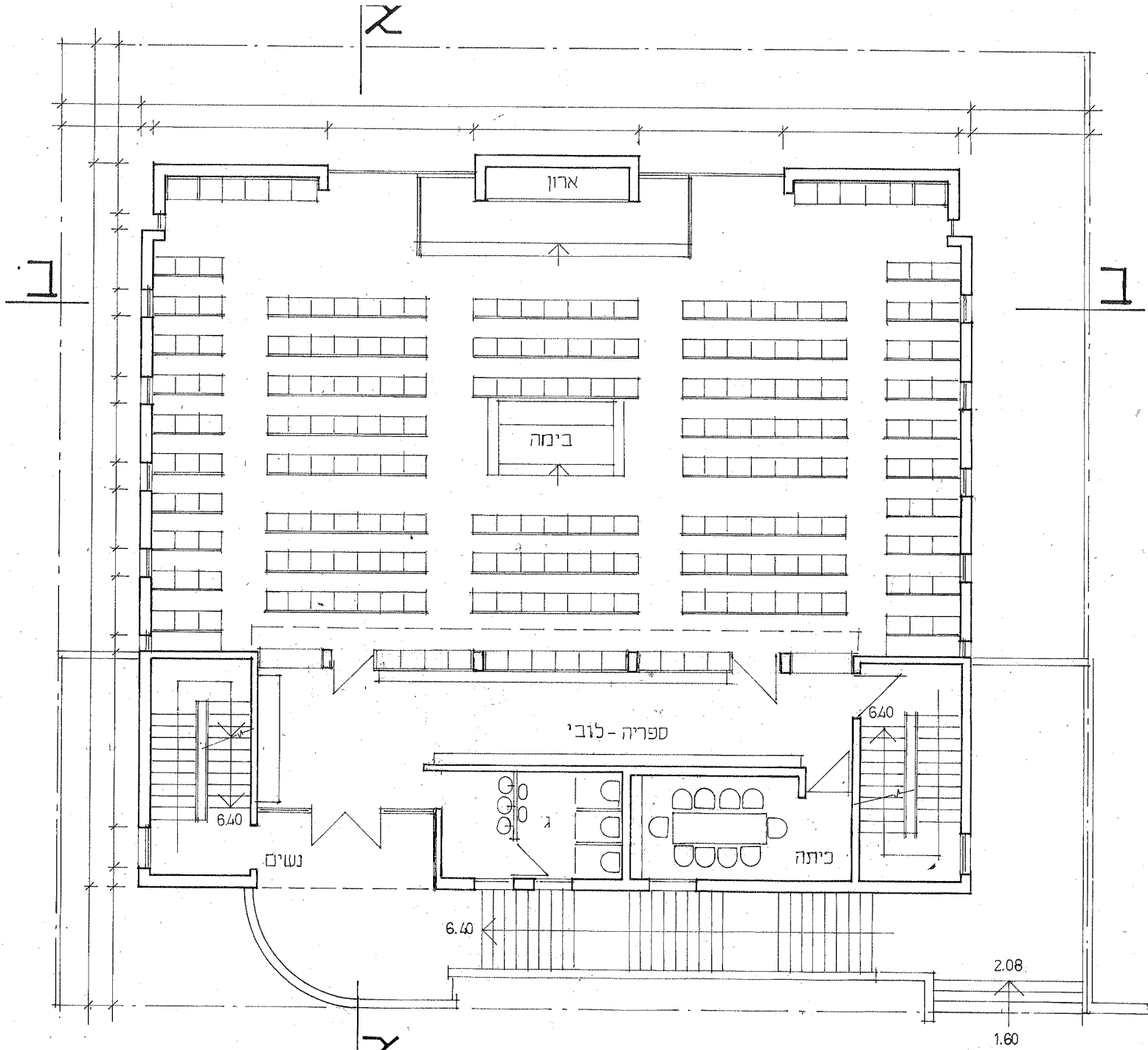
ASHKENAZI SYNAGOGUE קדמה עליונה ±6.40
