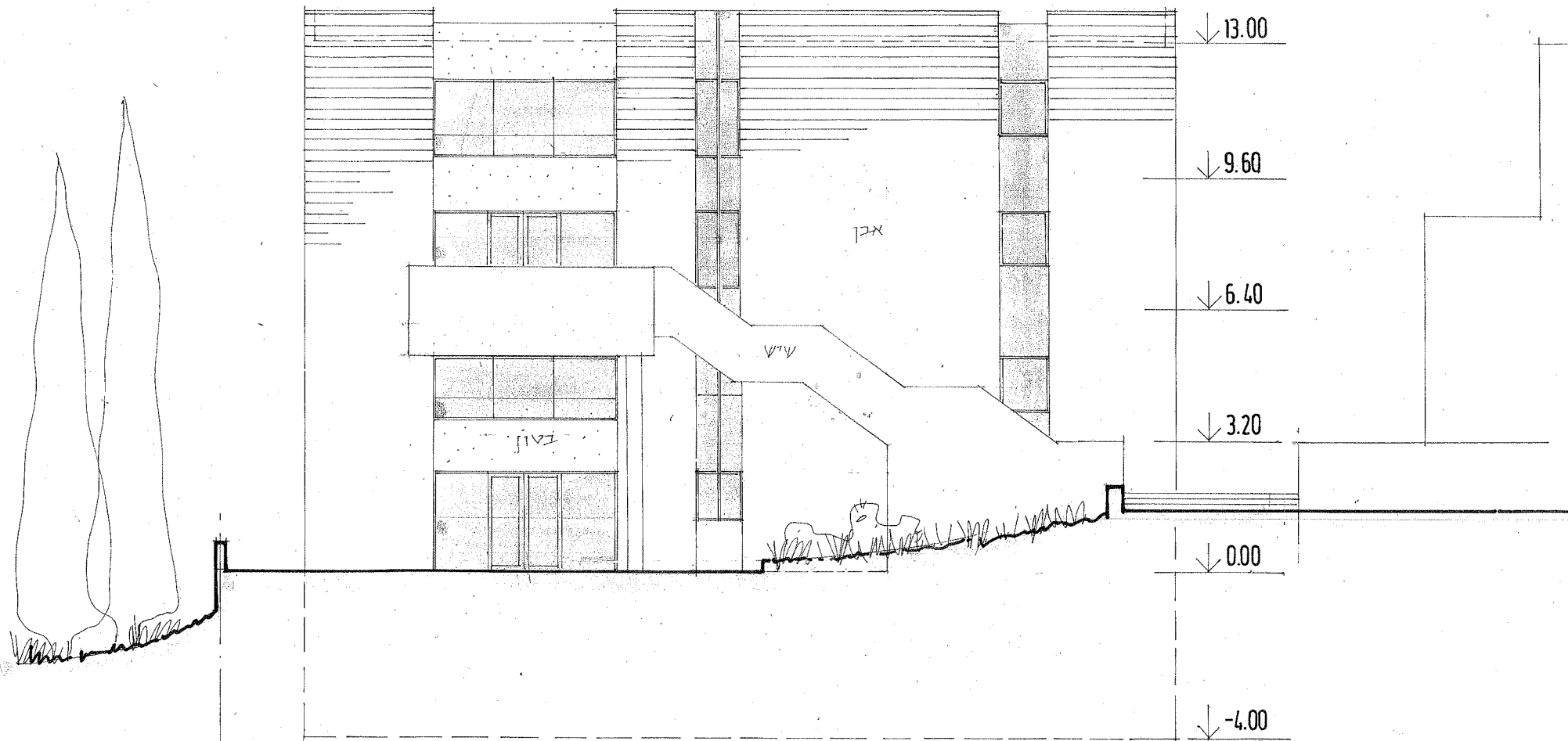
SOUTH ELEVATION חזית דרומית
